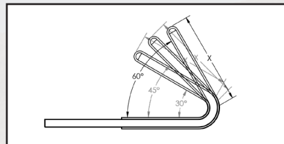
Side-Tension 30°, 45° & 60° Hooks
