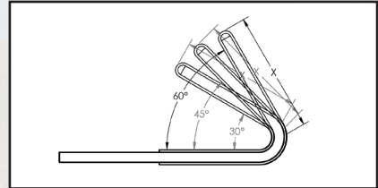
Side-Tension 30°, 45° & 60° Hooks
